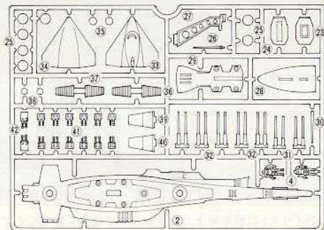
《部品図》
